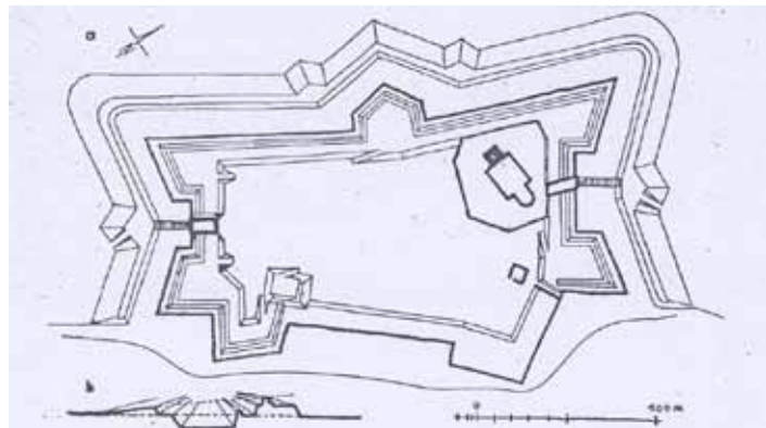
Ryc. Narys fortyfikacji bastionowych zamku w Dankowie. za: Janusz Bogdanowski, Twierdza z r. 1632 w Dankowie koło Krzepic. Arsenał. r. I. nr. 1. Kraków 1957. s. 89 i n. ryc. 18.
